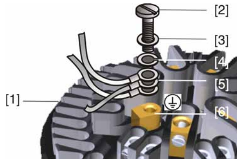
Kép 14: Védővezeték-csatlakozás
