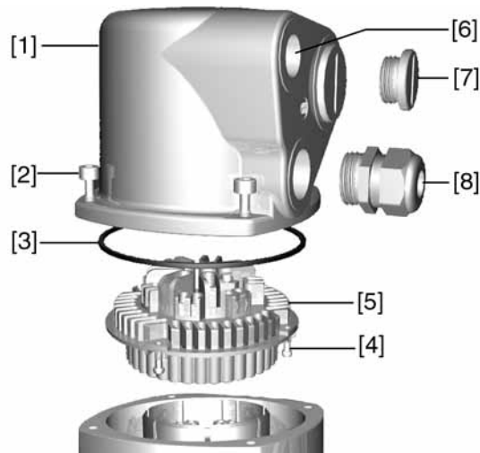
Kép 15: Példa: S kivitel
