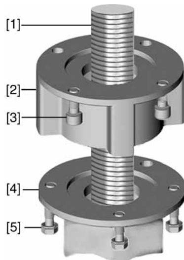
Kép 7: Szerelés "A" csatlakozóformával
