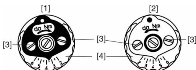
Kép 31: Nyomatékmérő fejek
