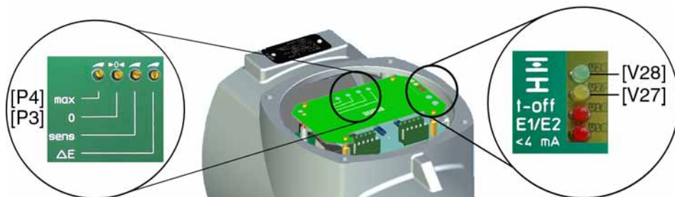
Kép 53: Helyzet szabályzó kártya
