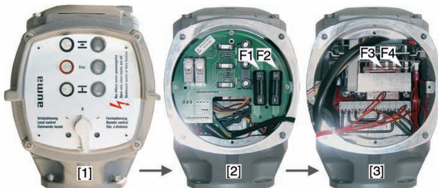
Kép 58: Hozzáférés a biztosítékokhoz
