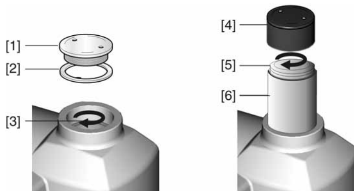
Kép 36: Üreges tengely/orsó
