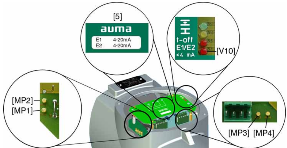
Kép 52: Helyszabályzó kártya
