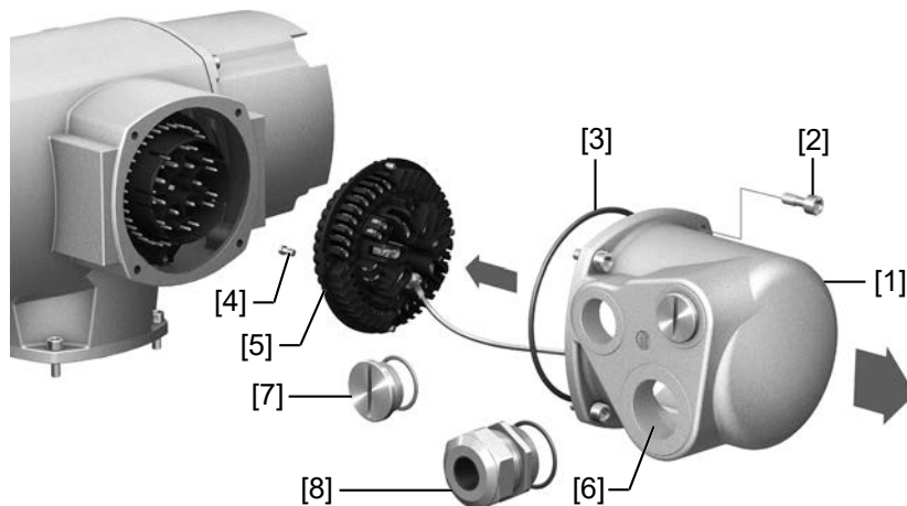
25. ábra: A csatlakozótér kinyitása
