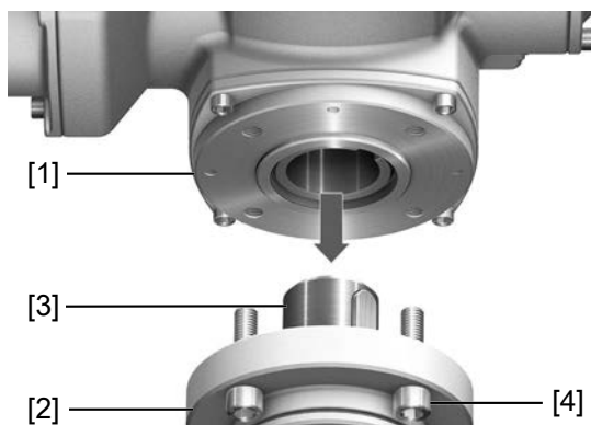
18. ábra: "B" csatlakozási forma szerelése
