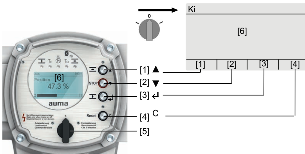
36. ábra: Helyi kezelőegység
