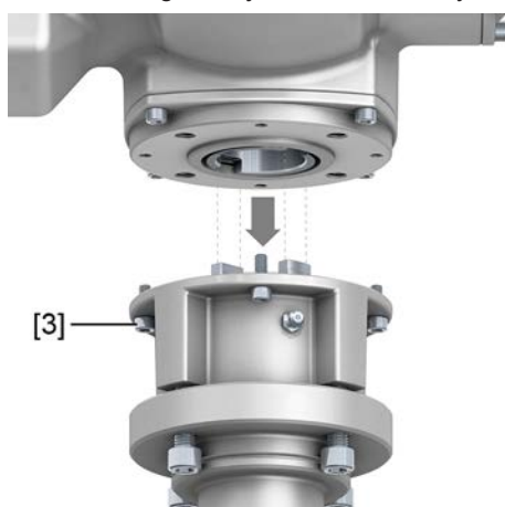
14. ábra: Forgató hajtómű a szerelvényorsóra
