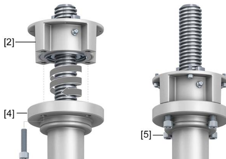
13. ábra: "A" szerelvénycsatlakozás orsón
