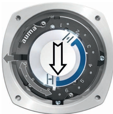
78. ábra: Leosztó áttétel beállítása
