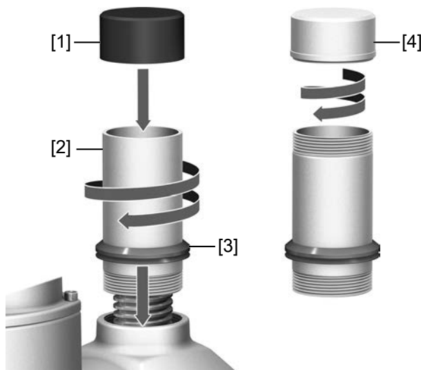
19. ábra: Orsóvédő cső szerelése
