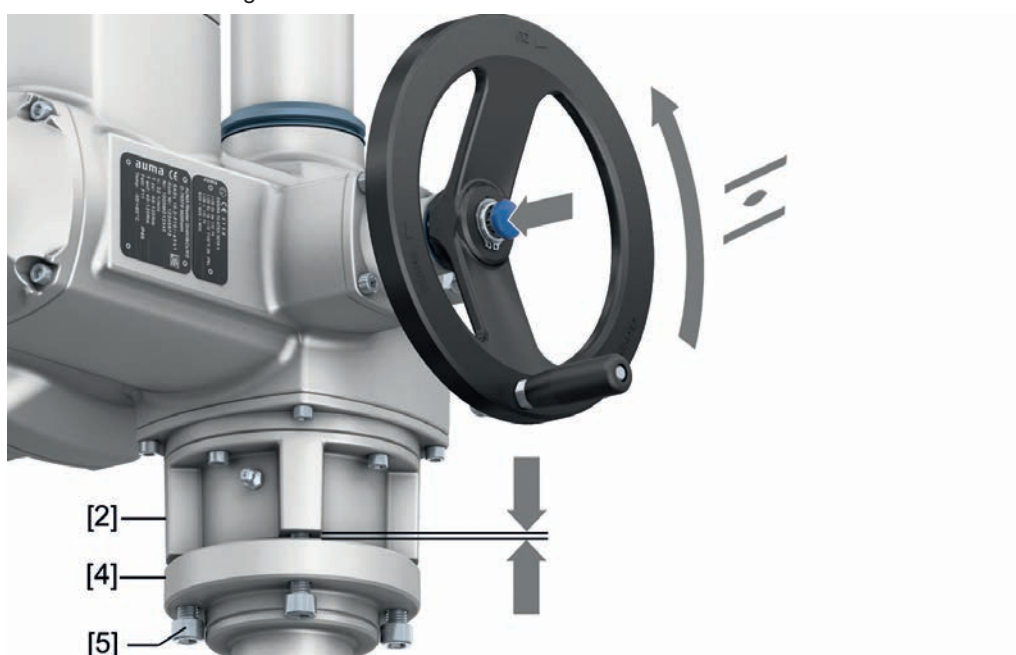
15. ábra: A karima meghúzása
