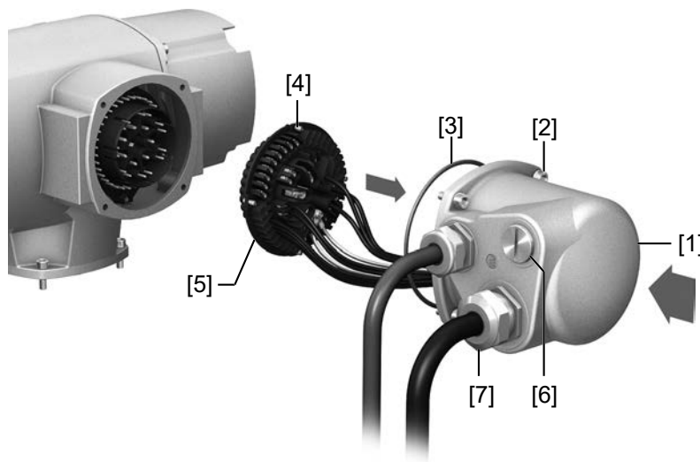
28. ábra: A csatlakozótér lezárása
