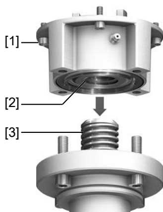
11. ábra: "A" csatlakozási forma felépítése
