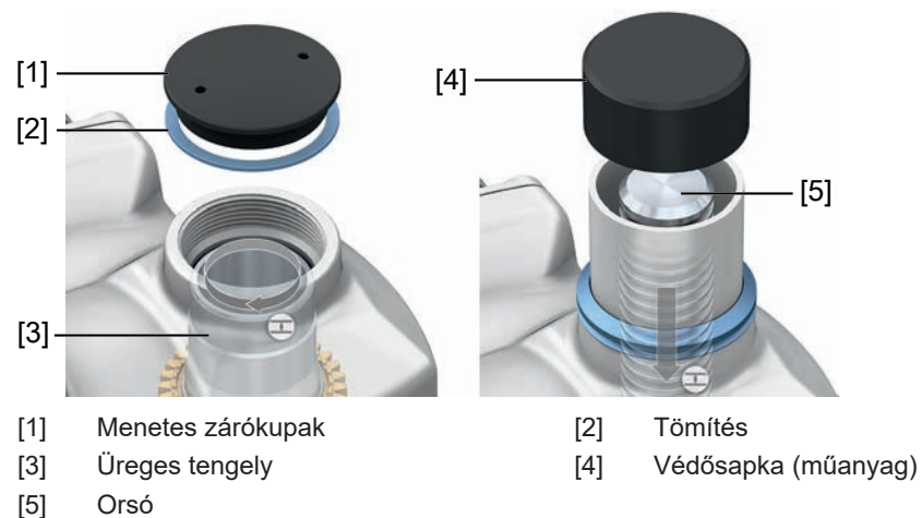
72. ábra: Az üreges tengely/orsó forgásirányának ellenőrzése ZÁR irányba történő járatásnál ( jobbra forgatva záró kivitel)
