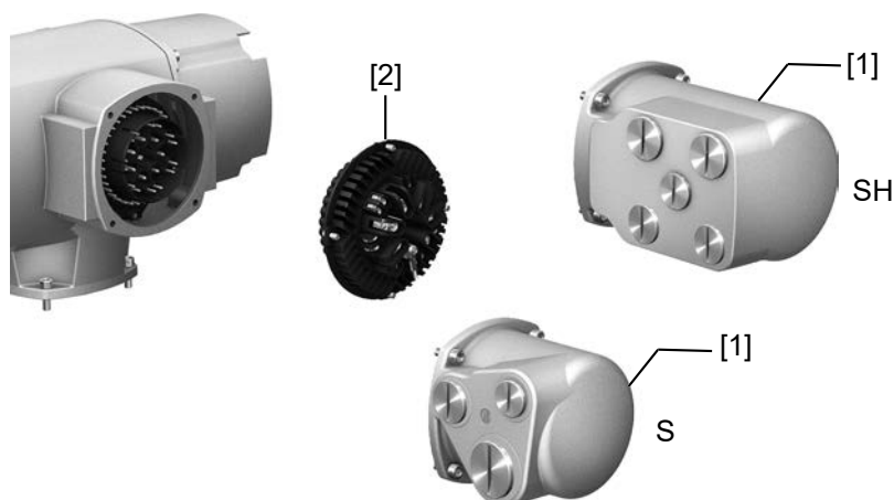
24. ábra: S és SH elektromos csatlakozó
