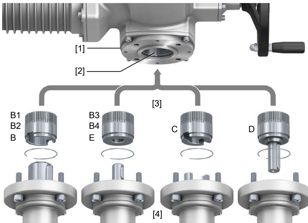
17. ábra: Szerelési elv
