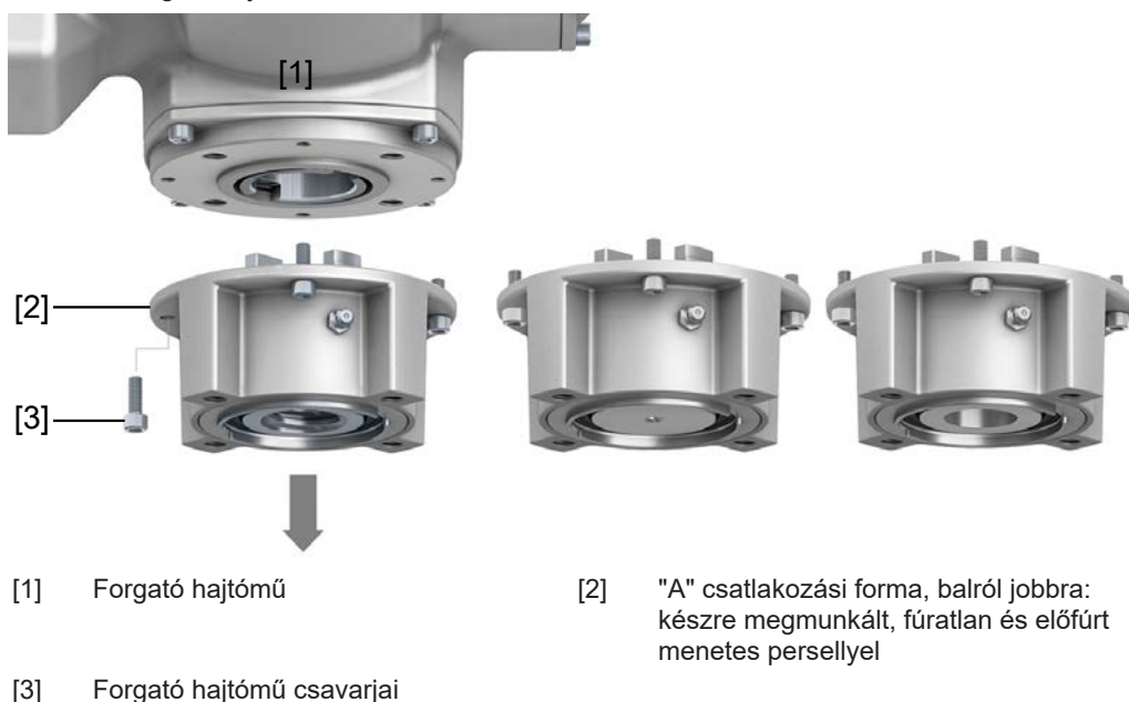
12. ábra: Forgató hajtómű "A" csatlakozási formával
