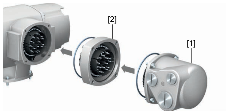
31. ábra: Elektromos csatlakozó DS közbenső kerettel
