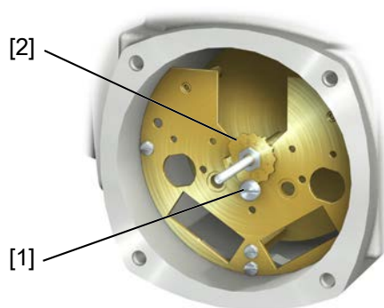
83. ábra: Vezérlőegység U-fokozóművel
