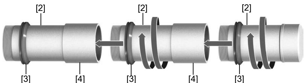
20. ábra: Részekből álló védőcső menetes karmantyúkkal (> 900 mm) (csak a 25.1 és 30.1 méretekre érvényes)
