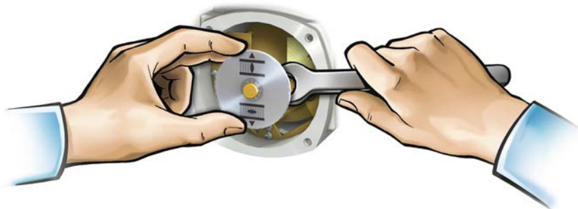
82. ábra: Helyzetjelző tárcsa lehúzása
