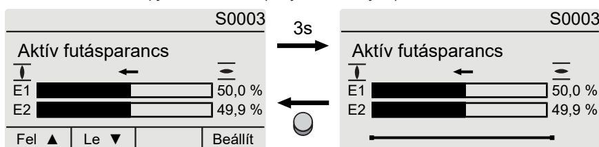
54. ábra: Jelzés alapjelvezérlésnél (helyzet szabályzó)
