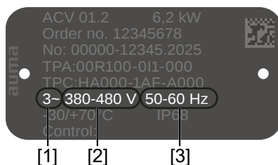
23. ábra: Példa a hajtómű-vezérlés típustáblájára
