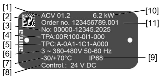
6. ábra: Hajtómű-vezérlés típusábra (példa)
