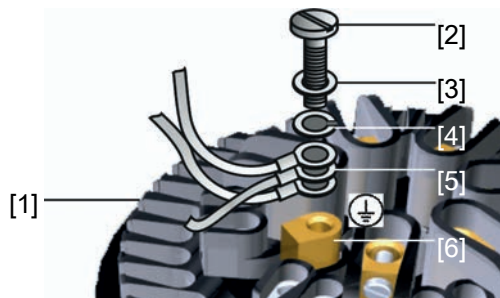
27. ábra: Védővezető csatlakozó
