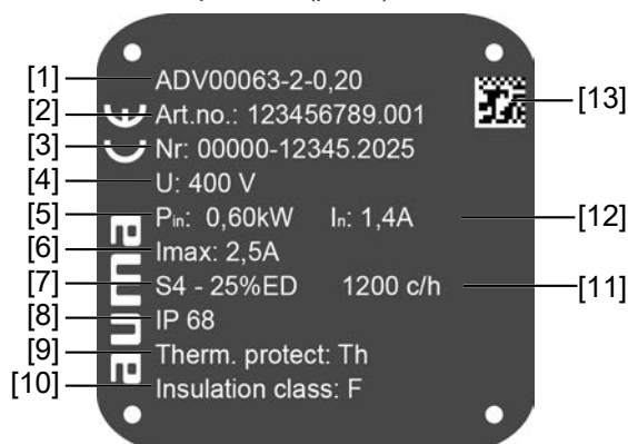
7. ábra: Motor típusábra (példa)
